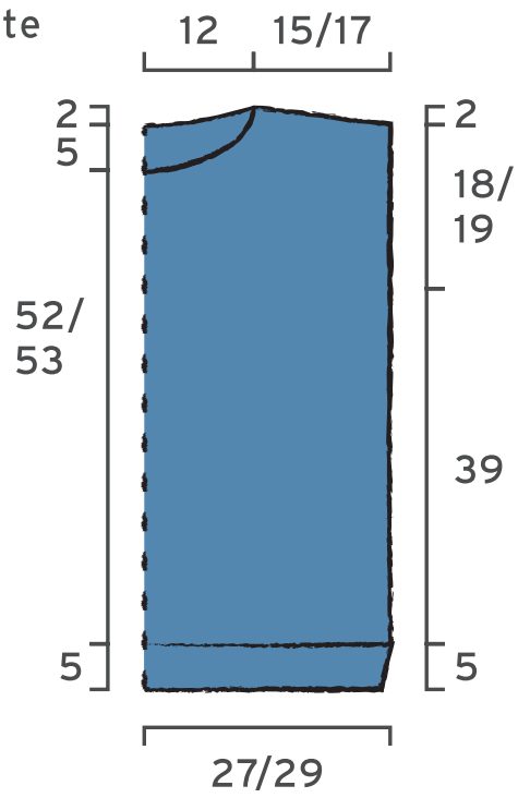
Ärmel, Hälfte
